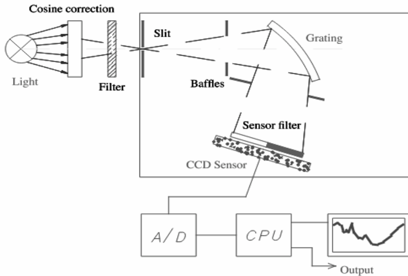
Schemat systemu spektrometrycznego
