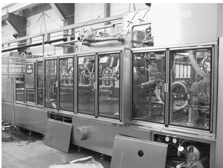
Rys. 3. Widok znacznej części automatu typ 100 od tyłu
